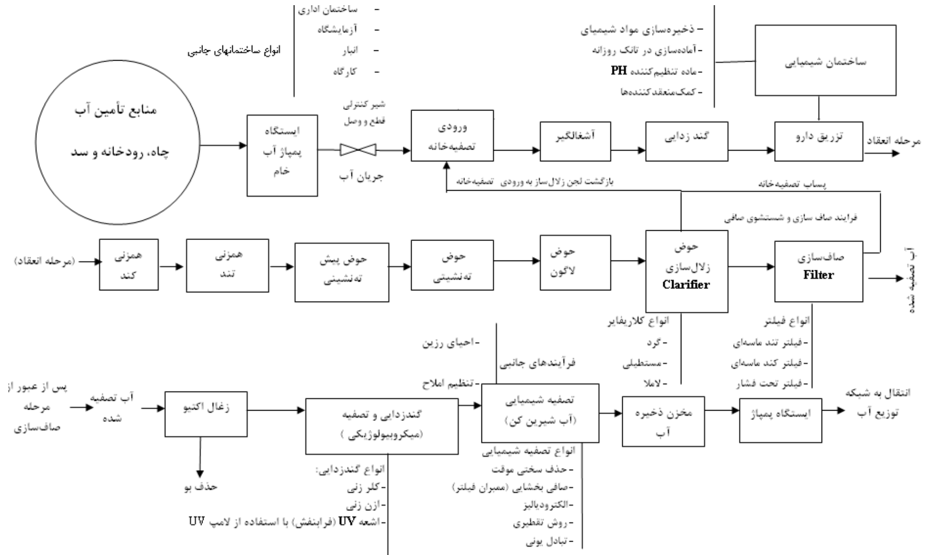
شکل (۱۲-۱) - مدل شماتیک فرآیندهای تصفیه آب
